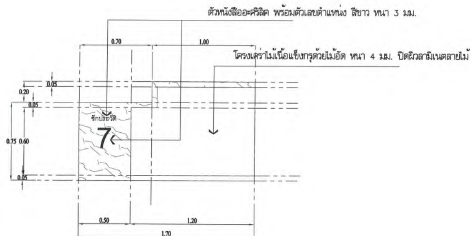
แบบรูปด้าน 1 SCALE 1:25
