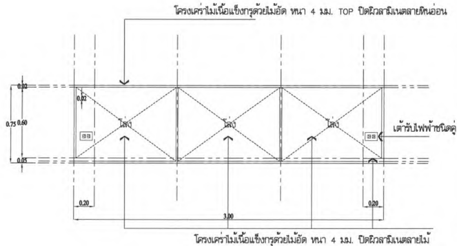
แบบรูปด้าน 2 SCALE 1:25
