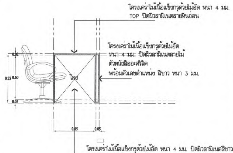
แบบรูปตัด A SCALE 1:25
