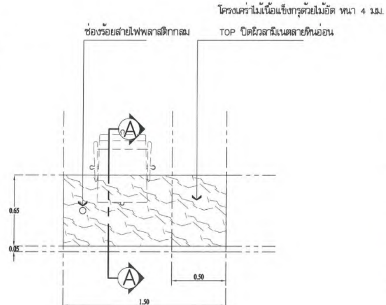
แบบแปลน BLN-01 SCALE 1:25
