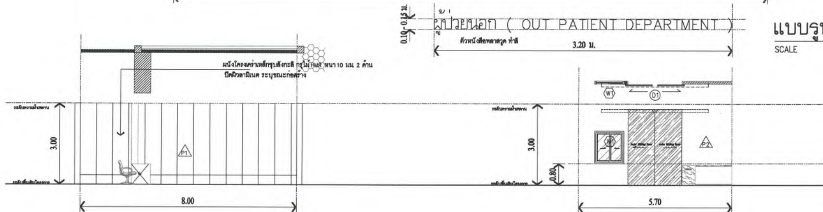
แบบรูปด้านที่ 3 SCALE 1 : 100
