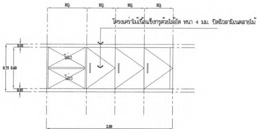
แบบรูปด้าน ① SCALE 1:25
