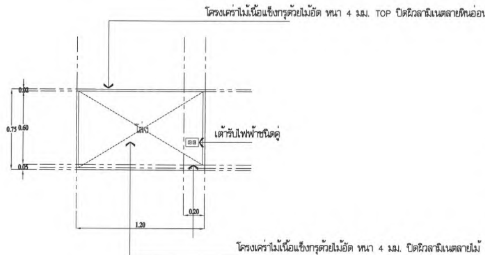
แบบรูปด้าน ② SCALE 1:25
