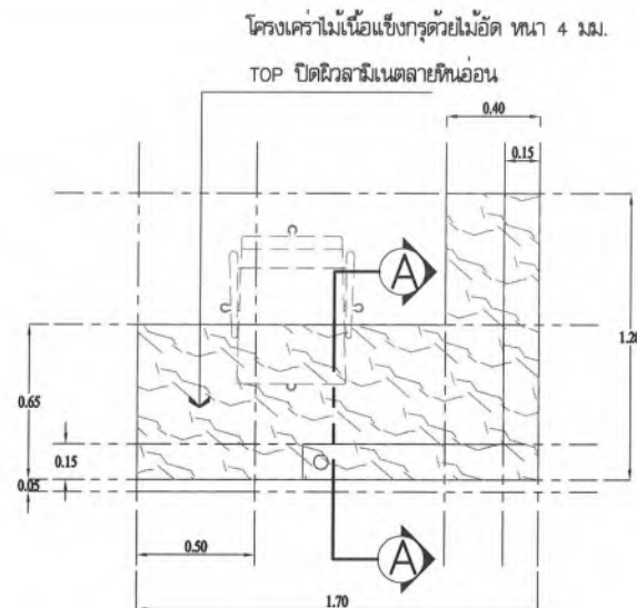
แบบแปลน BLN-03 SCALE 1:25
