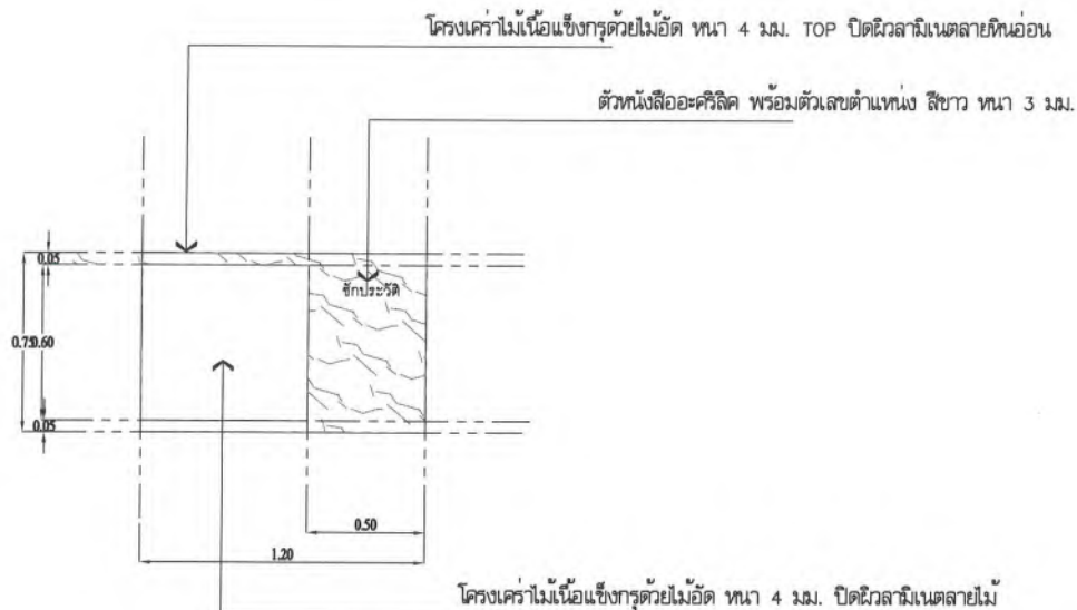
แบบรูปด้าน ① SCALE 1:25
