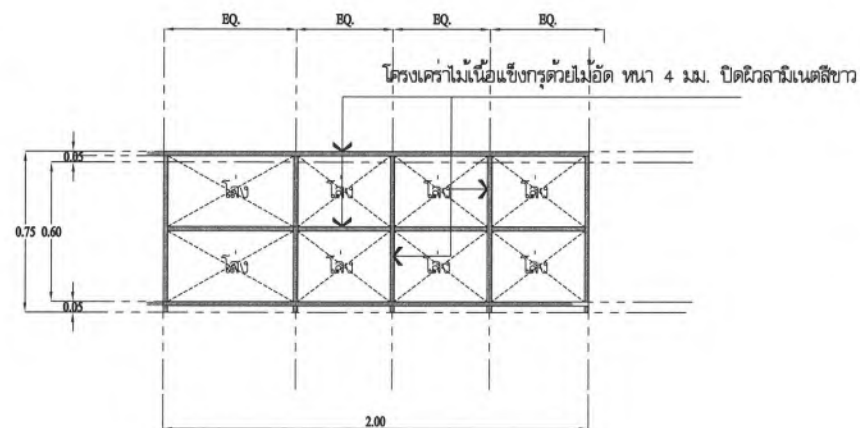
แบบรูปตัด A SCALE 1:25
