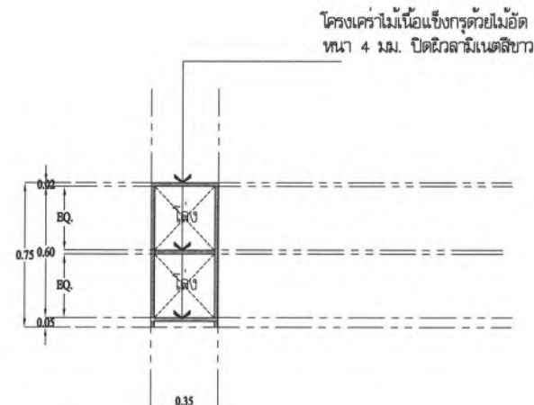
แบบรูปตัด A SCALE 1:25
