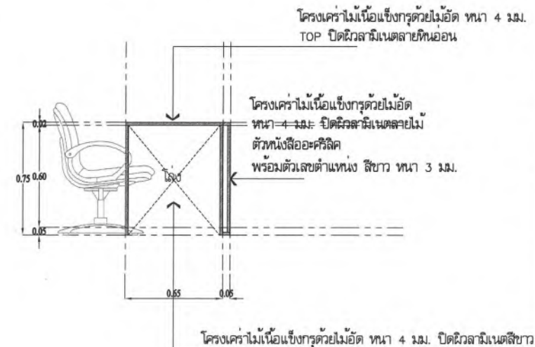
แบบรูปตัด A SCALE 1:25
