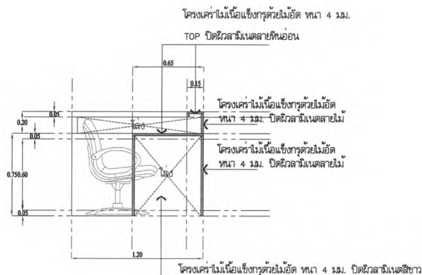
แบบรูปตัด A SCALE 1:25
